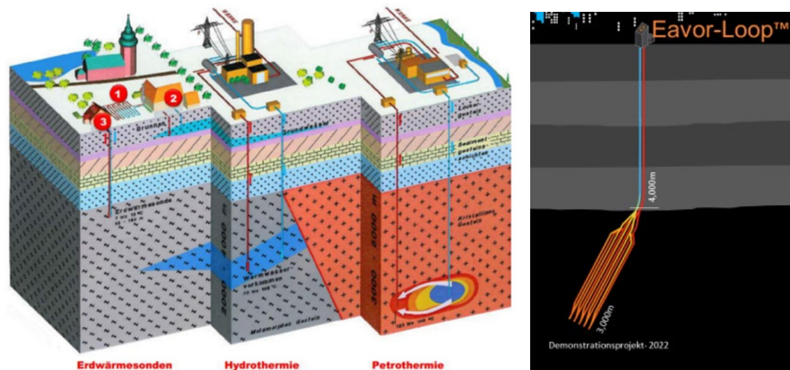
Abbildung 9: Schematische Darstellung von Nutzungssystemen für Geothermie (linke Seite) 30 und des Eavor-Loops (rechte Seite) 31
