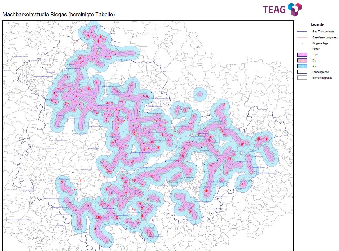
Abbildung 18: Darstellung von Biogasanlagen und der Erdgasinfrastruktur der TEN Thüringer Energienetze GmbH 105
