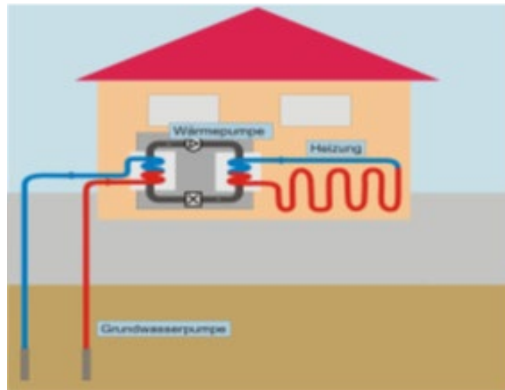
Abbildung 5: Funktionsschema - Anlagen mit Grundwasserpumpen 22
