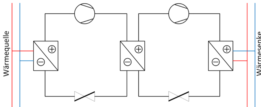
Abbildung 21: Zweistufiger Wärmepumpenkreislauf 187
