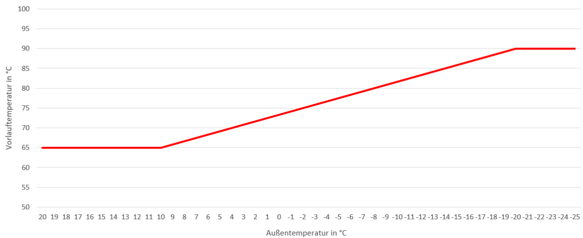
Abbildung 26: Temperaturfahrkurve HKW Schwarza für das Fernwärmenetz Bad Blankenburg
