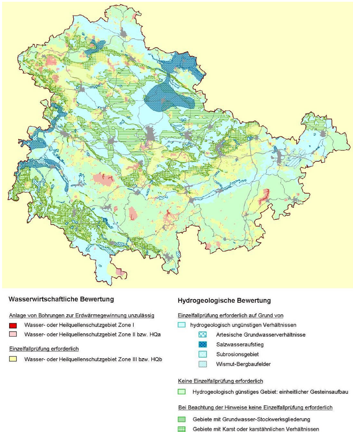
Abbildung 7: Übersichtskarte zur Geothermie in Thüringen 28
