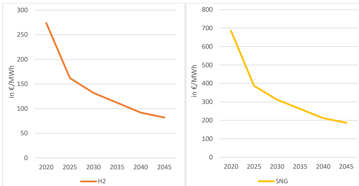
Abbildung 17: Zu Grunde gelegter Preispfad für Wasserstoff und SNG
